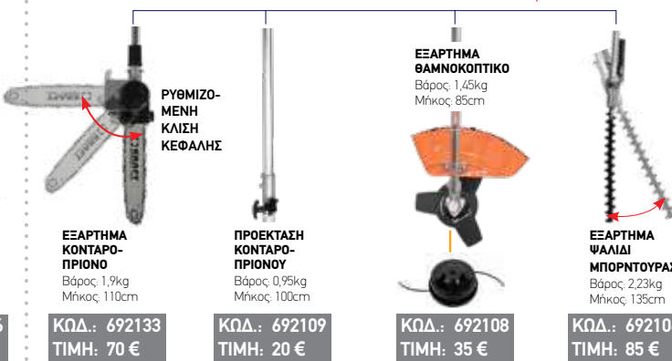
ΕΞΑΡΤΗΜΑ ΨΑΛΙΔΙ ΜΠΟΡΝΤΟΥΡΑΣ Βάρος: 2,23kg Μήκος: 135cm
